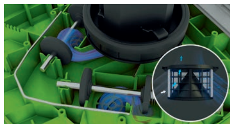
Filterreiniging door het omkeren van de luchtstroom
